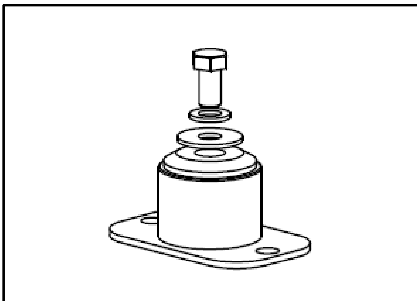
圖1)檢查附件是否齊全，避震器有無缺陷破損。
